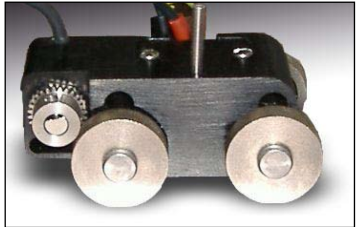
Mini B-Scan Magnetic Wheel Encoder
